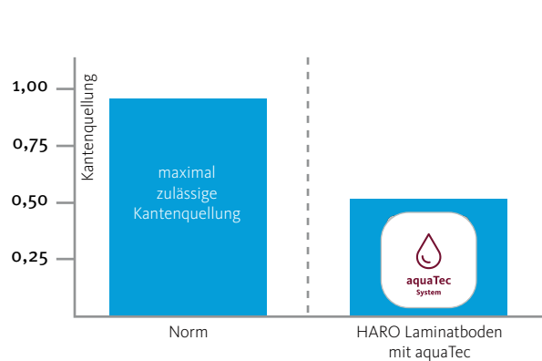
Kantenquellung von Laminatböden bei Wassereinfluss
