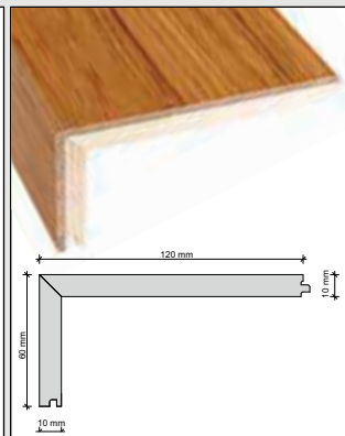
Treppenabschlussleiste mit beidseitiger Verbindung Trittstufe: 120 mm Setzstufe: 60 mm
