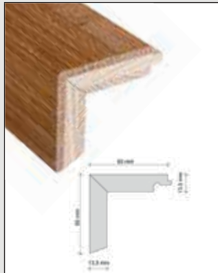
Treppenabschlussleiste mit einseitiger Verbindung Trittstufe: 60 mm Setzstufe: 60 mm
