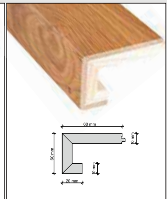
Treppenabschlussleiste eingeschlagen Trittstufe: 60 mm Setzstufe: 40 mm Einschlag: 20 mm
