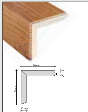
Treppenabschlussleiste mit einseitiger Verbindung Trittstufe: 60 mm Setzstufe: 60 mm
